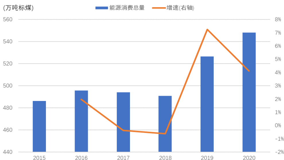
图 1 2015—2020 年遂宁市能源消费总量及增速
